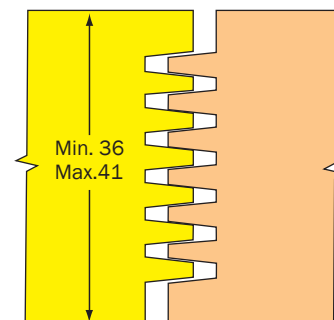
Med sex koniska notskivor
