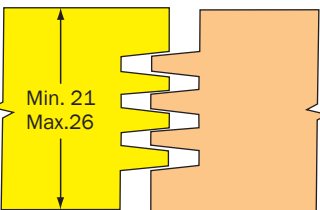
Med tre koniska notskivor
