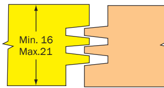
Med två koniska notskivor
