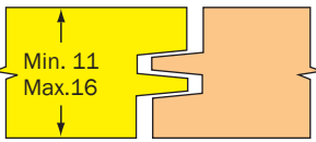
Med en konisk notskiva
